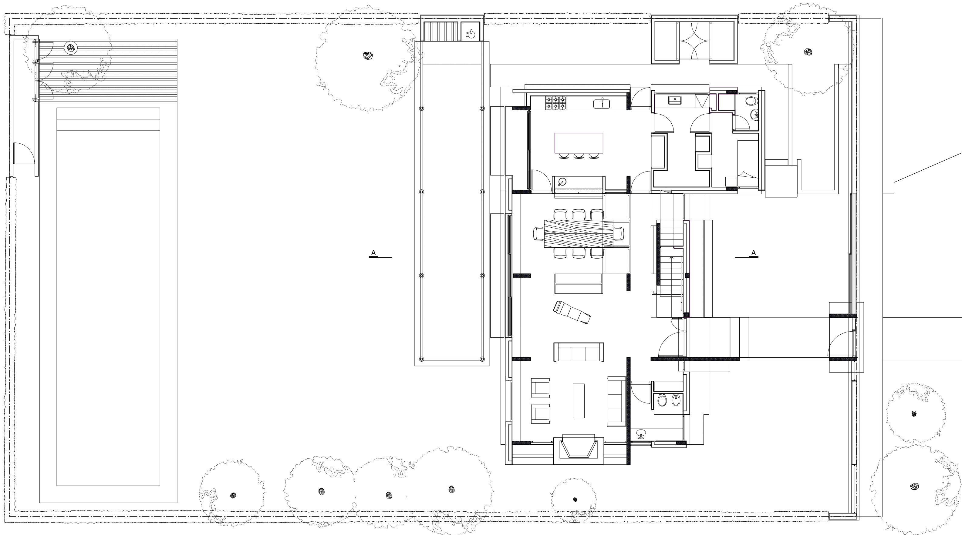
PLANTA BAJA
