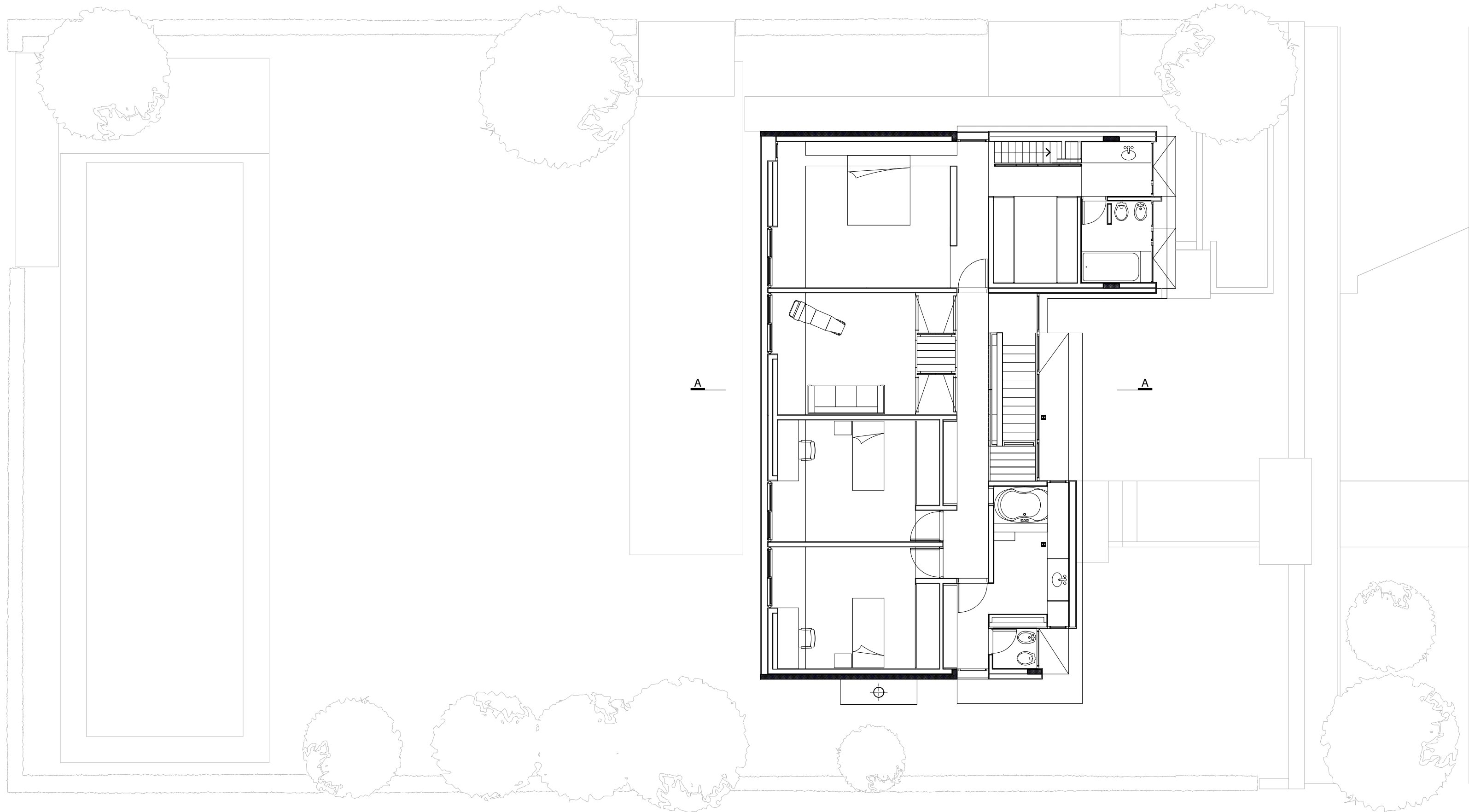
PLANTA ALTA
