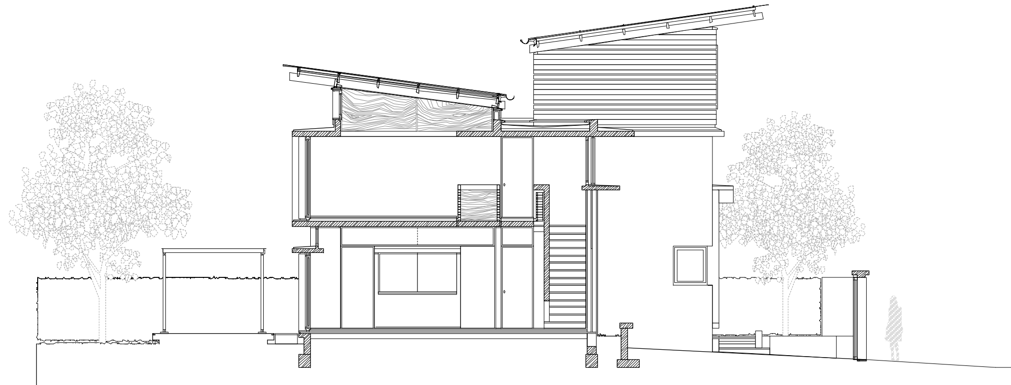
CORTE A
