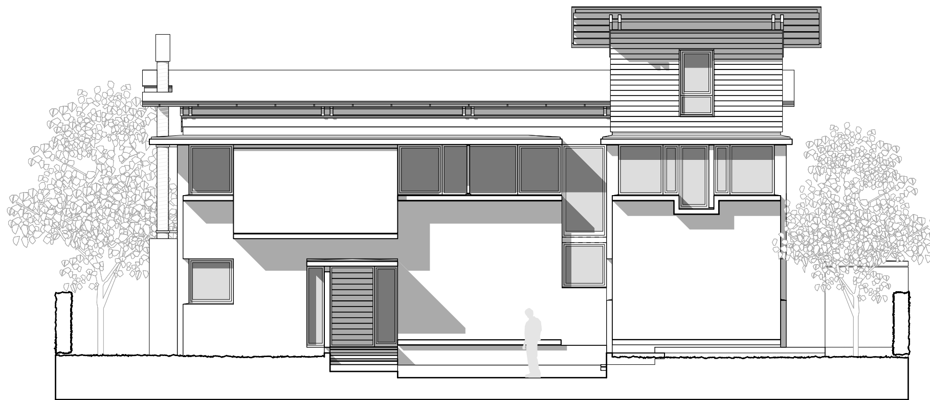
VISTA FRENTE
