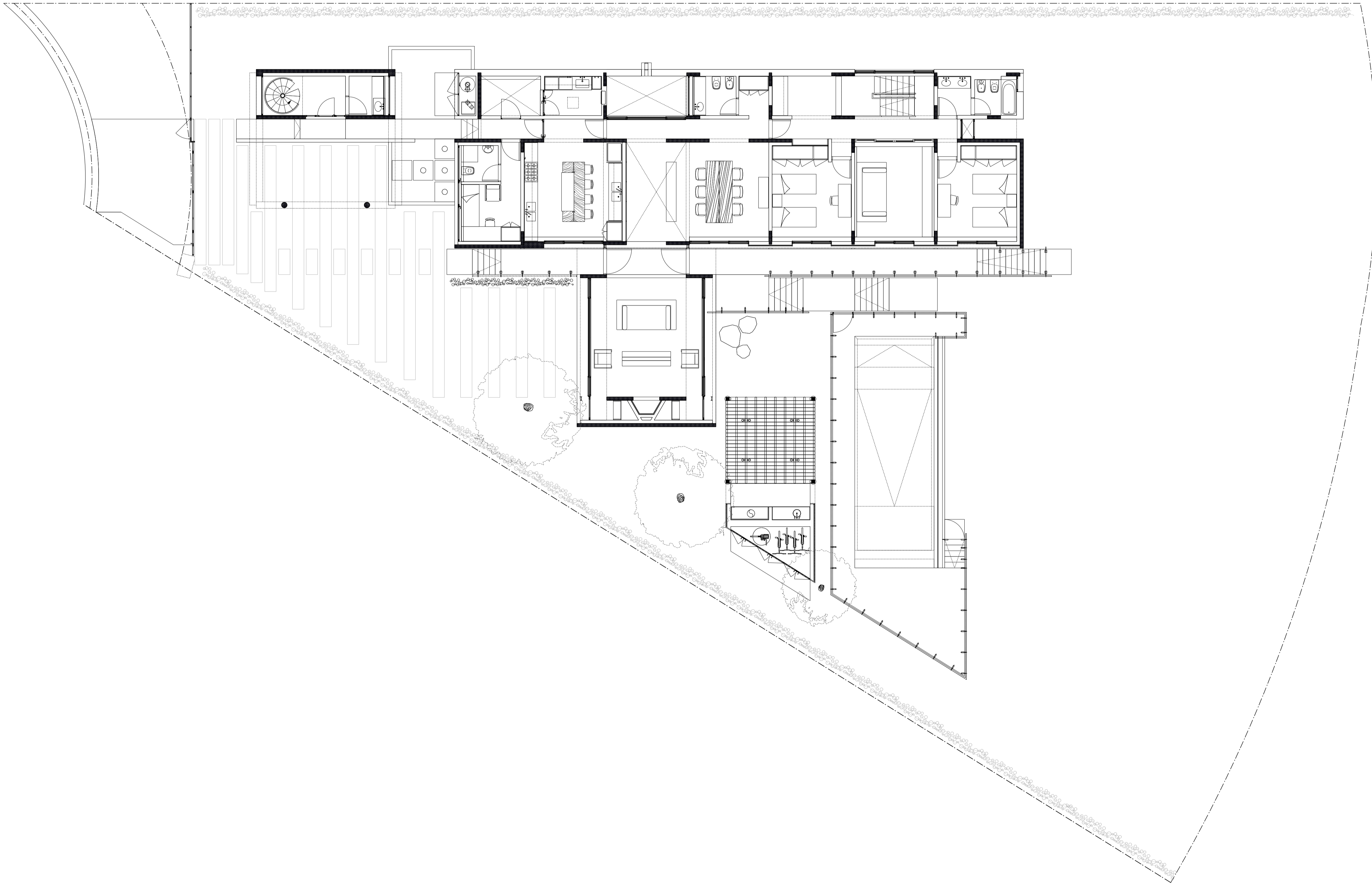
PLANTA BAJA
